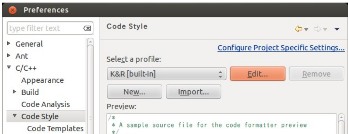
図 2.1: Code Style
